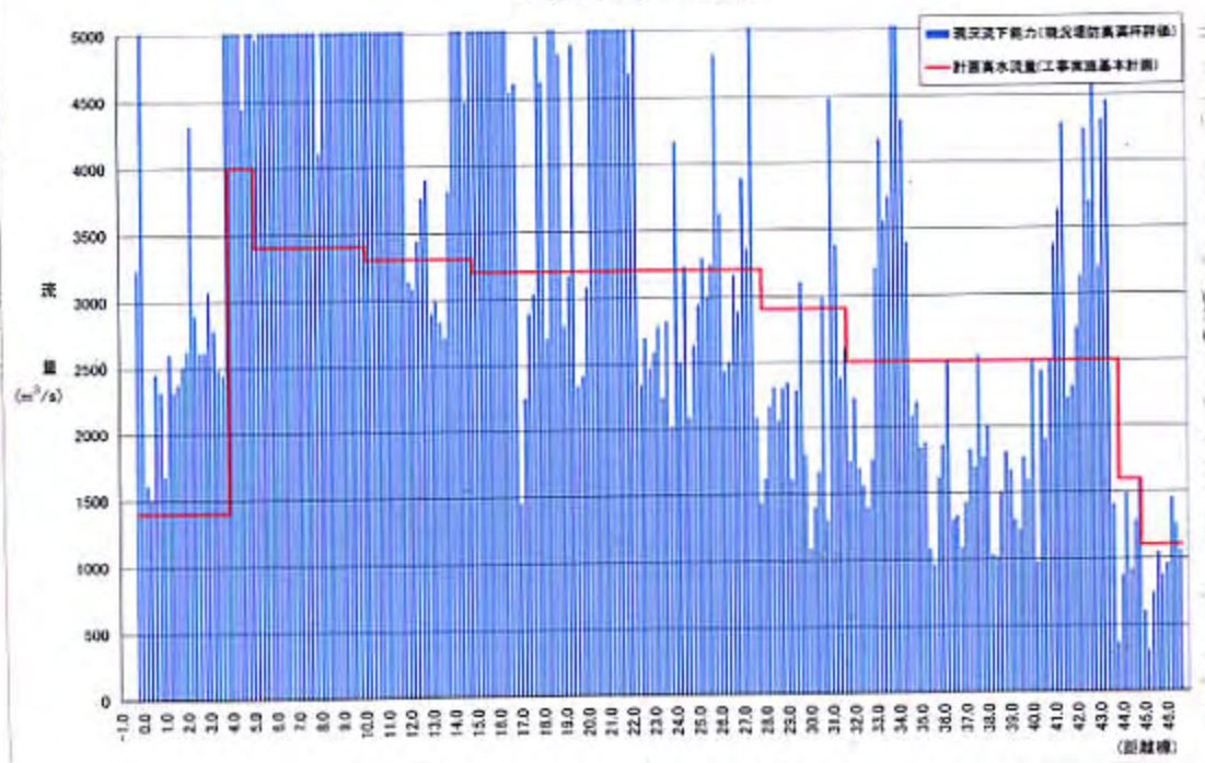
揖保川:現況流下能力図
