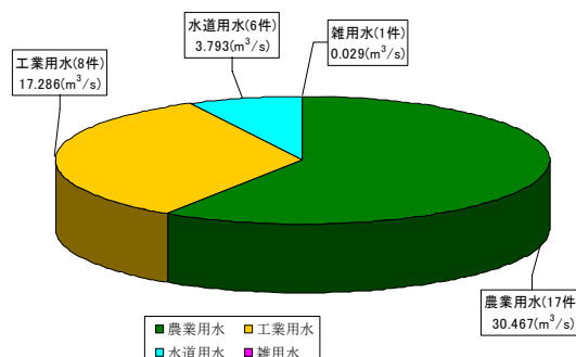
図-2.2.2 加古川利水状況
