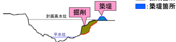
図-4.1.12 滝野・多井田地区 (その2) の河川整備イメージ
