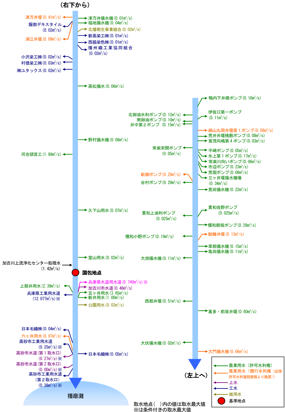
図-2.2.3 加古川水系水利模式図
