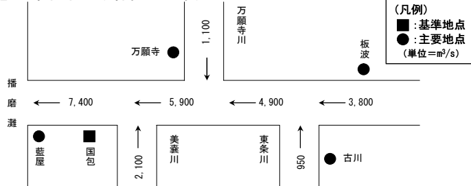
図-1.2.3 各計画における流量配分図
