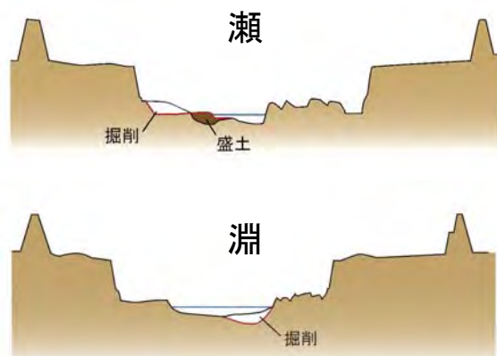
図－4.3.1 掘削イメージ（瀬・淵）
