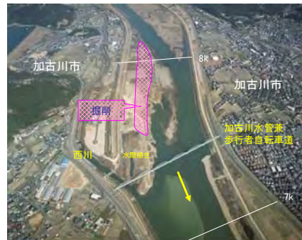
図-4.1.4 平荘地区 (その1) の河川整備イメージ
