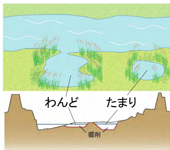
図－4.3.2 掘削イメージ（わんど・たまり）
