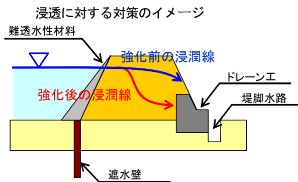
図-4.1.17 堤防の安全性確保（質的整備）に関するイメージ
