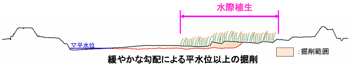
図-4.3.4 掘削イメージ（水際植生）
