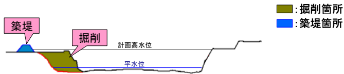
図-4.1.13 おいだ 多井田地区の河川整備イメージ
