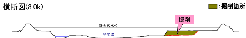
図-4.1.5 平荘地区 (その2) の河川整備イメージ
