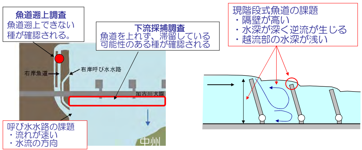
図-4.3.6 加古川大堰における魚道の課題
