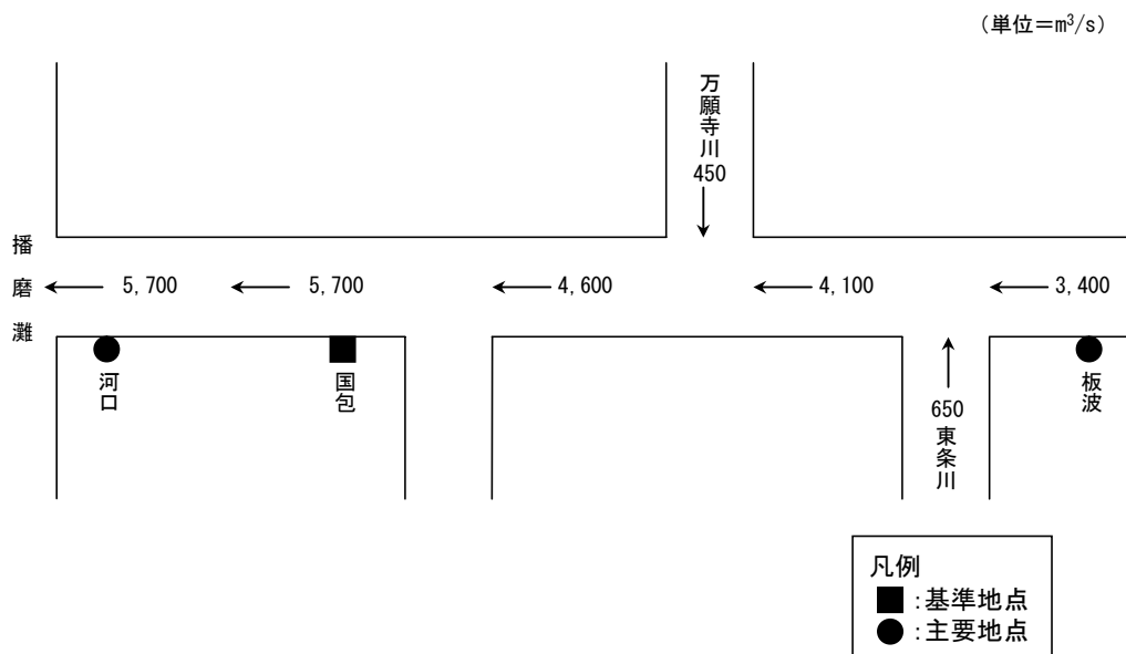
図-3.1.2 河川整備において目標とする流量
