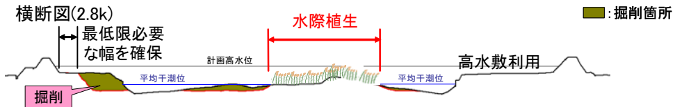
図-4.1.3 古新地区の河川整備イメージ
