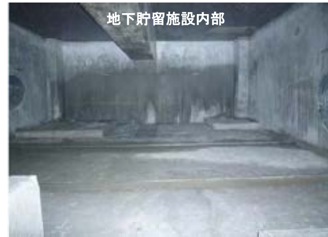
雨水貯留浸透施設の事例 【横浜市内】
