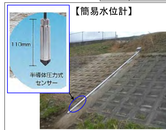
CCTV・簡易水位計設置状況
