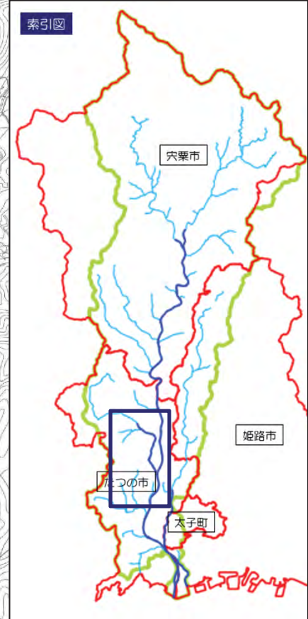
揖保川水系栗栖川洪水浸水想定区域図 （家屋倒壊等氾濫想定区域（氾濫流））
