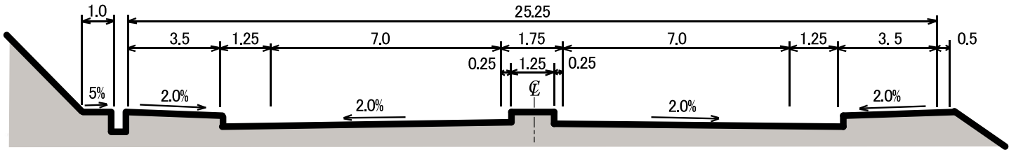
一般部（歩道なし）
