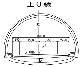
トンネル部
