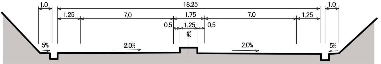
一般部（歩道なし）
