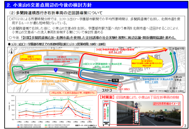
▲迂回誘導によるソフト対策の検討事例
