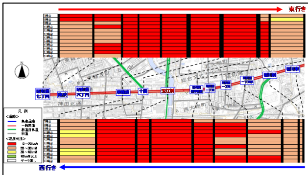
▲交差点周辺の速度状況把握
