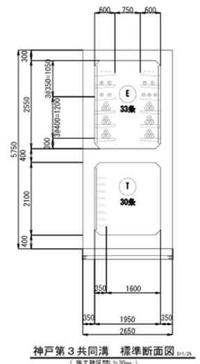
標準断面図
