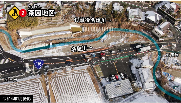
名塩川の付け替え及び橋の架設工事を行っています。
