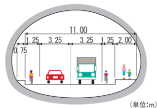
【標準断面：トンネル部】
