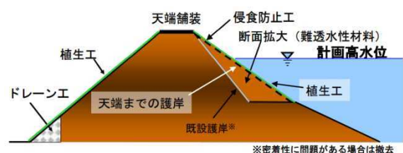
図 4.3.2-4 堤防強化対策工法の例
