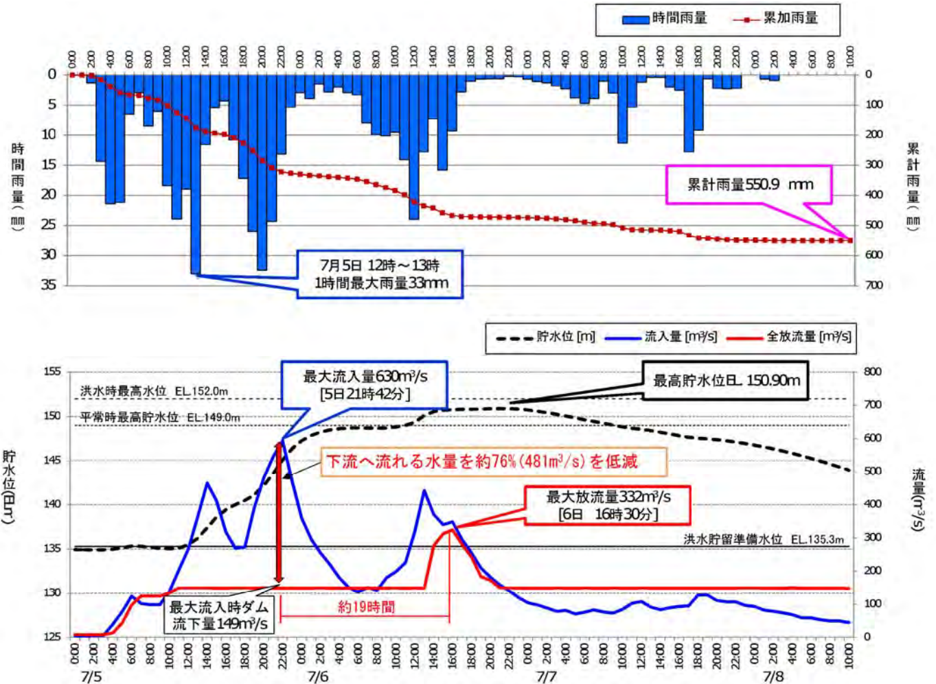
平成30年7月豪雨 一庫ダム防災操作図
