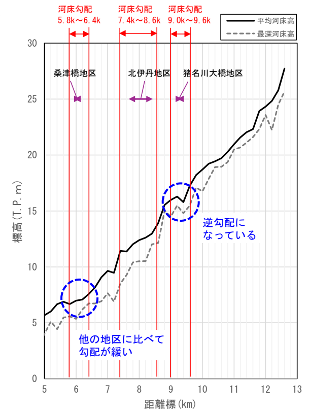
対象区間の縦断図 (R2河道)
