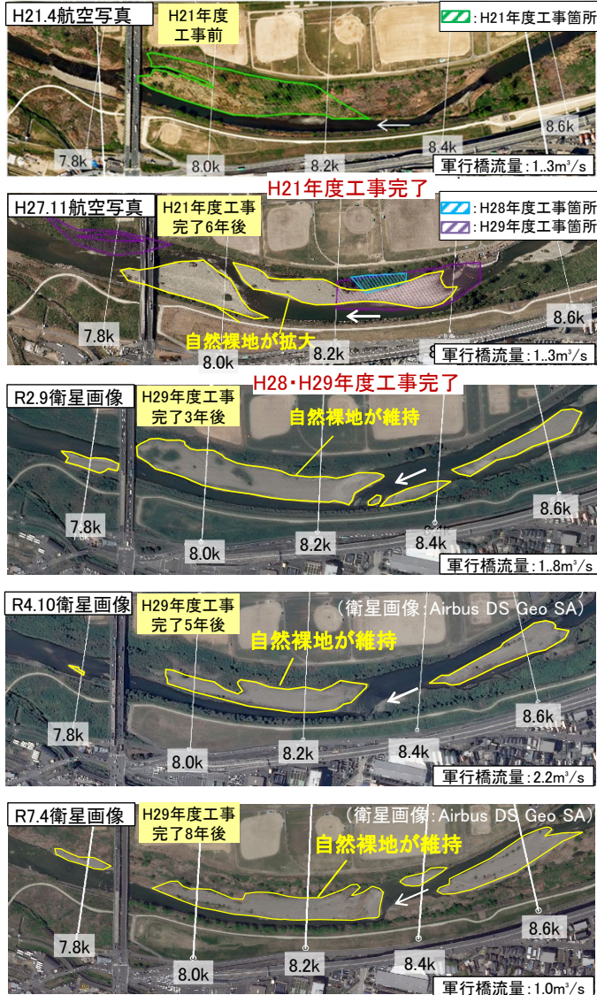
北伊丹地区周辺の航空写真と工事箇所平面図(5時点)
