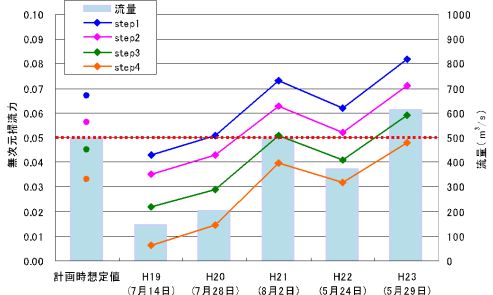
年最大流量時の無次元掃流力の推移 〔6.6k 地点〕
