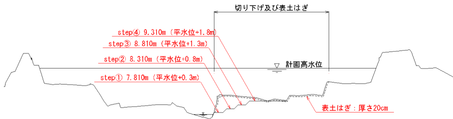
試験施工箇所の横断面図
