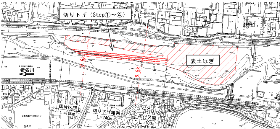
試験施工箇所の平面図
