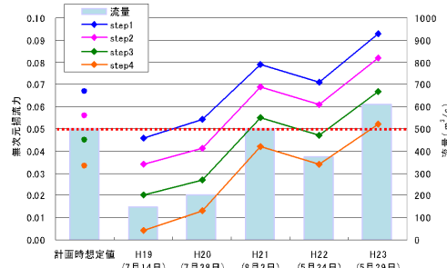
年最大流量時の無次元掃流力の推移 〔6.8k 地点〕
