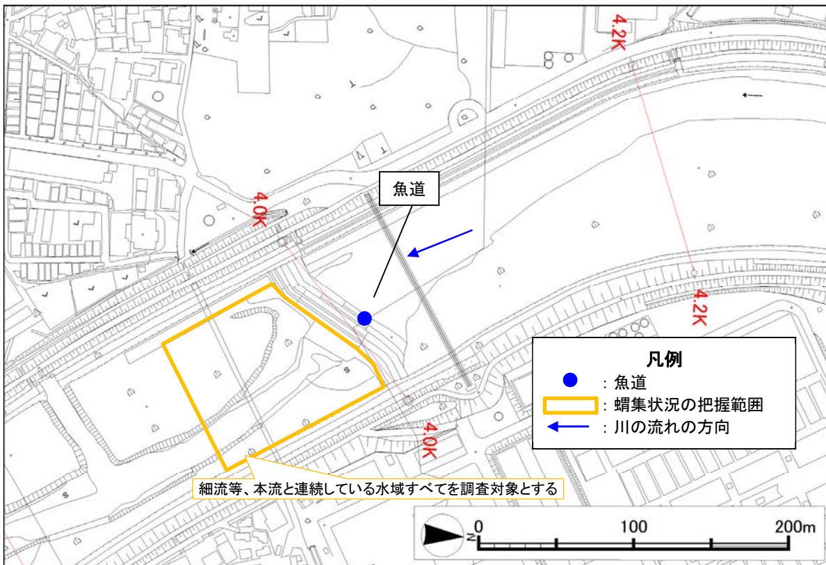
図 3.2-2 (1) 蜻集状況の把握範囲 [淀藻猪 1 (大井井堰)]
