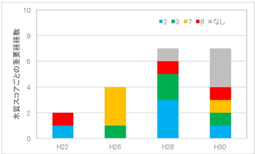
9 図 3.3-3 底生動物重要種の水質スコア別の出現状況の変遷（猪名川(底)-3）
