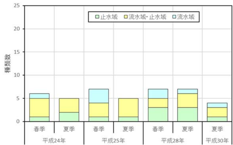
3 図 3.3-2 湿地群落を指標するトンボ目（ヤゴ類）の生息環境別確認種数の変遷（猪名川(底)-1）
