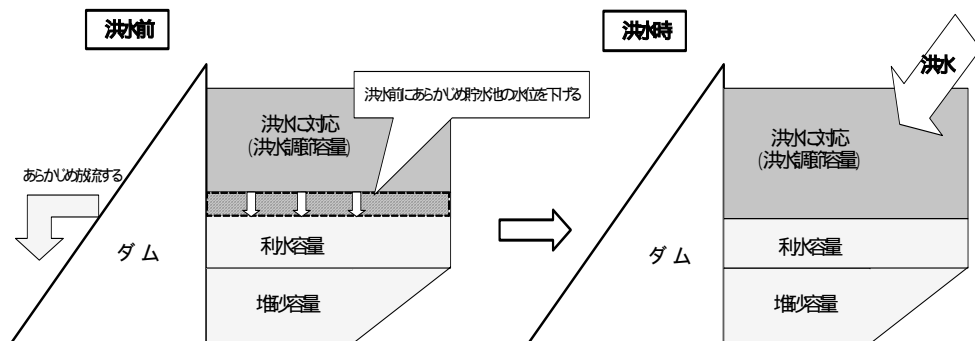
予備放流イメージ図
