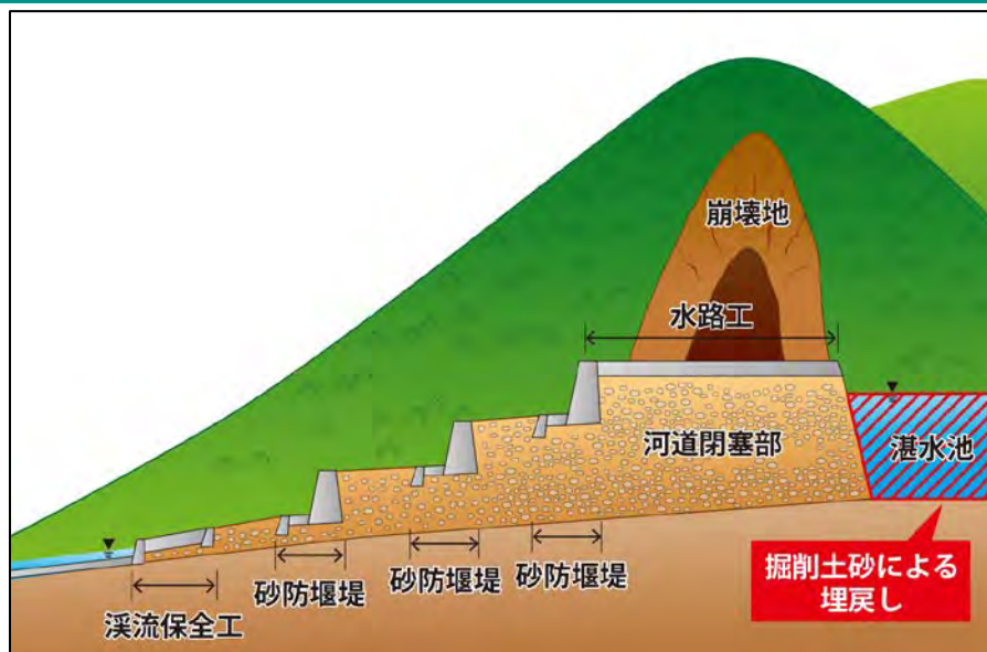
図 11 河道閉塞対策
