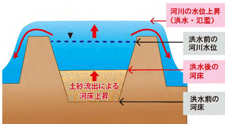
図 14 土砂流出による河床上昇で発生する洪水氾濫のイメージ
