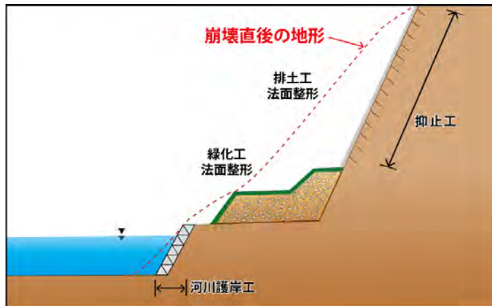
図 12 斜面对策
