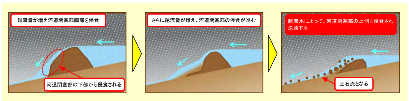
図8 崩壊過程（越流侵食）
