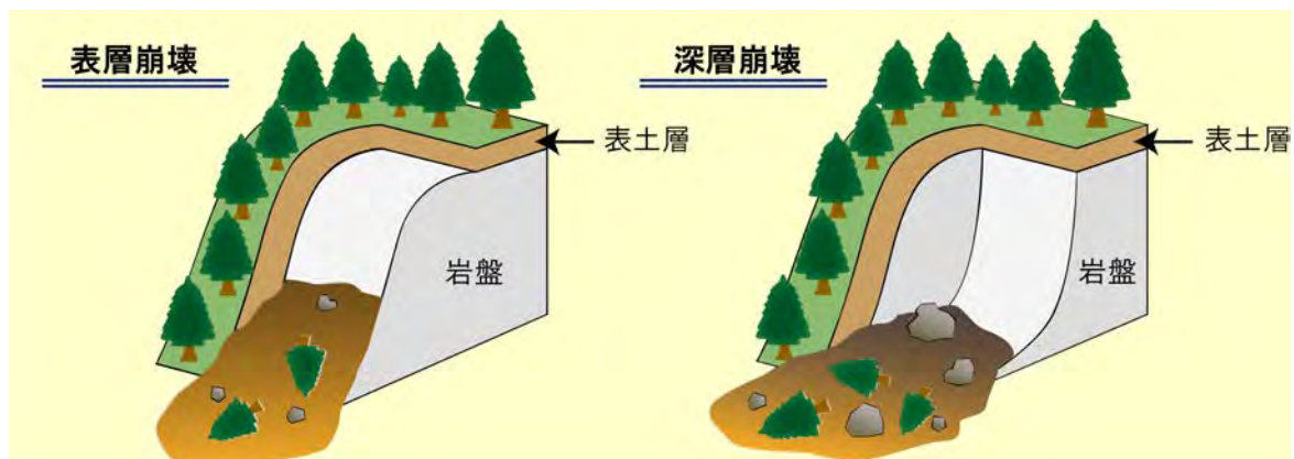
図7 表層崩壊と深層崩壊の違い
