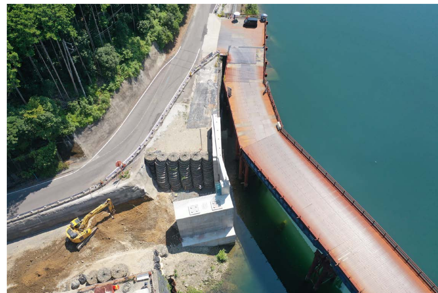
② 北山村下尾井(道路改良・1号橋)
