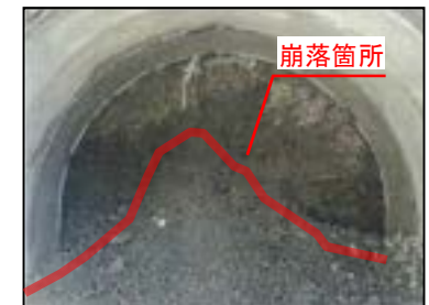
<トンネル内崩落状況写真>
