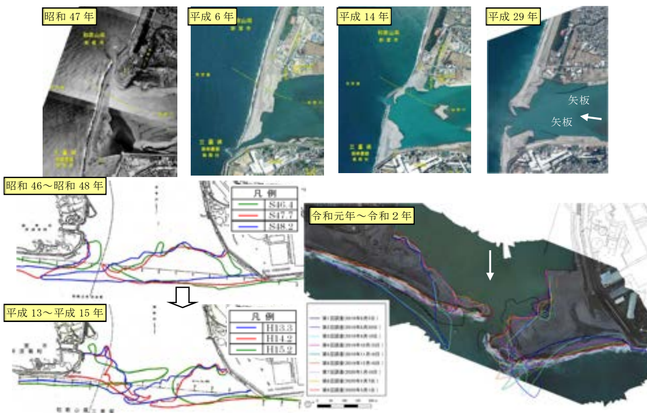
図-2.18 熊野川河口部砂州の経年変化
