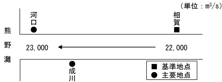
図－3.2 熊野川流量配分図
