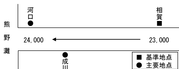
熊野川計画高水流量図 (単位：m 3 /s)
