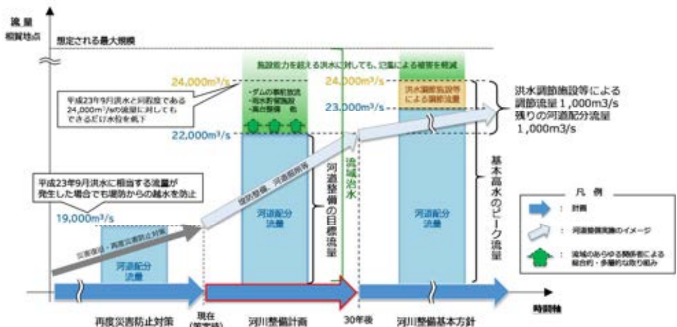
図－3.3 新宮川水系河川整備基本方針の目標に向けた段階的な整備イメージ図
