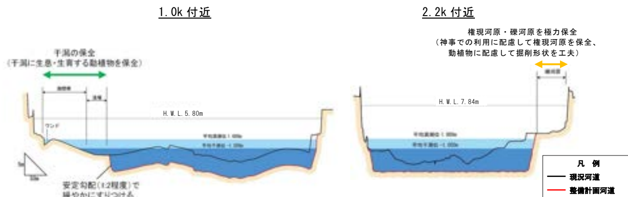
図－4.2 河道掘削イメージ（横断図）
