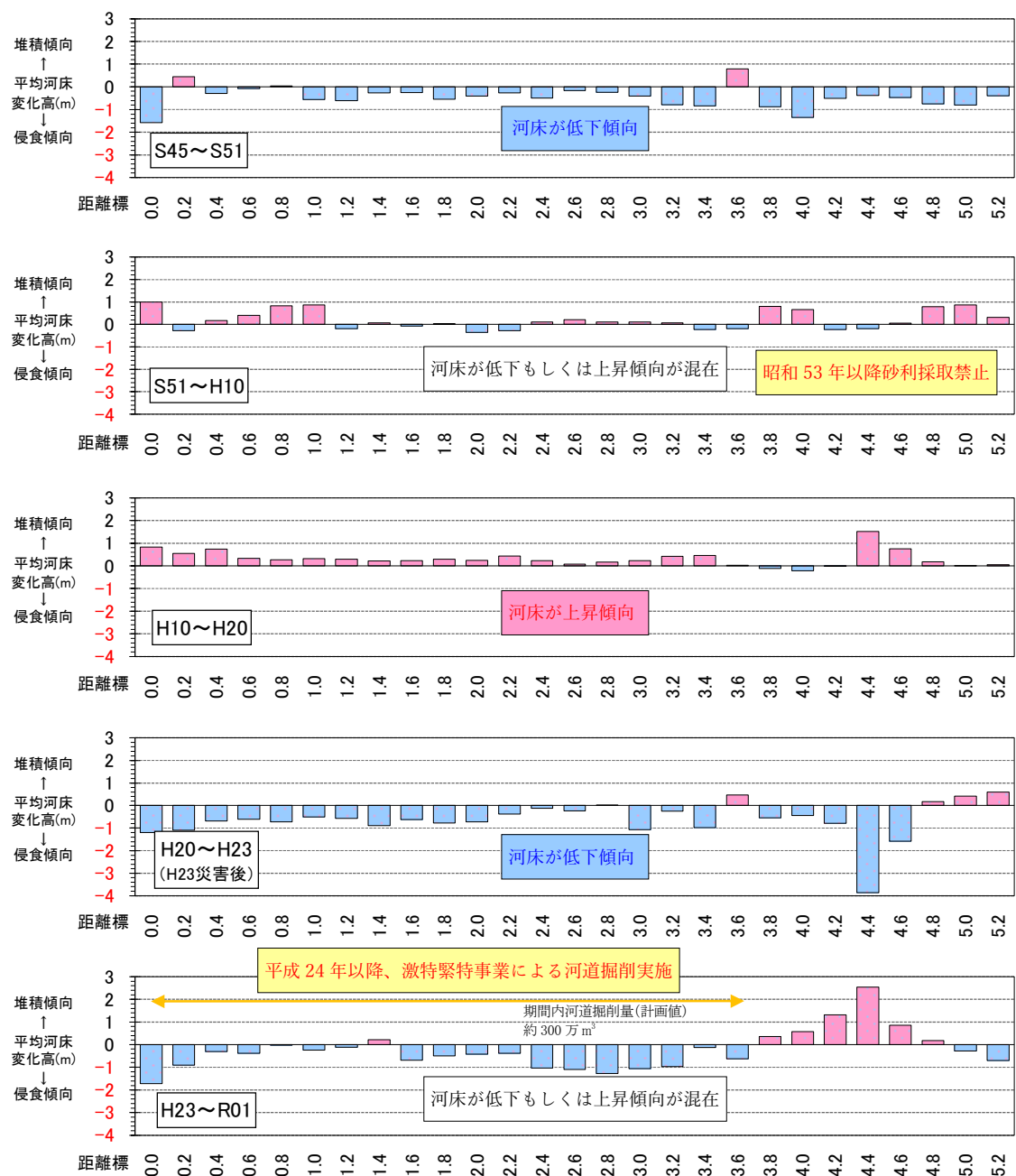
図－2.14 国管理区間の平均河床の変動量
