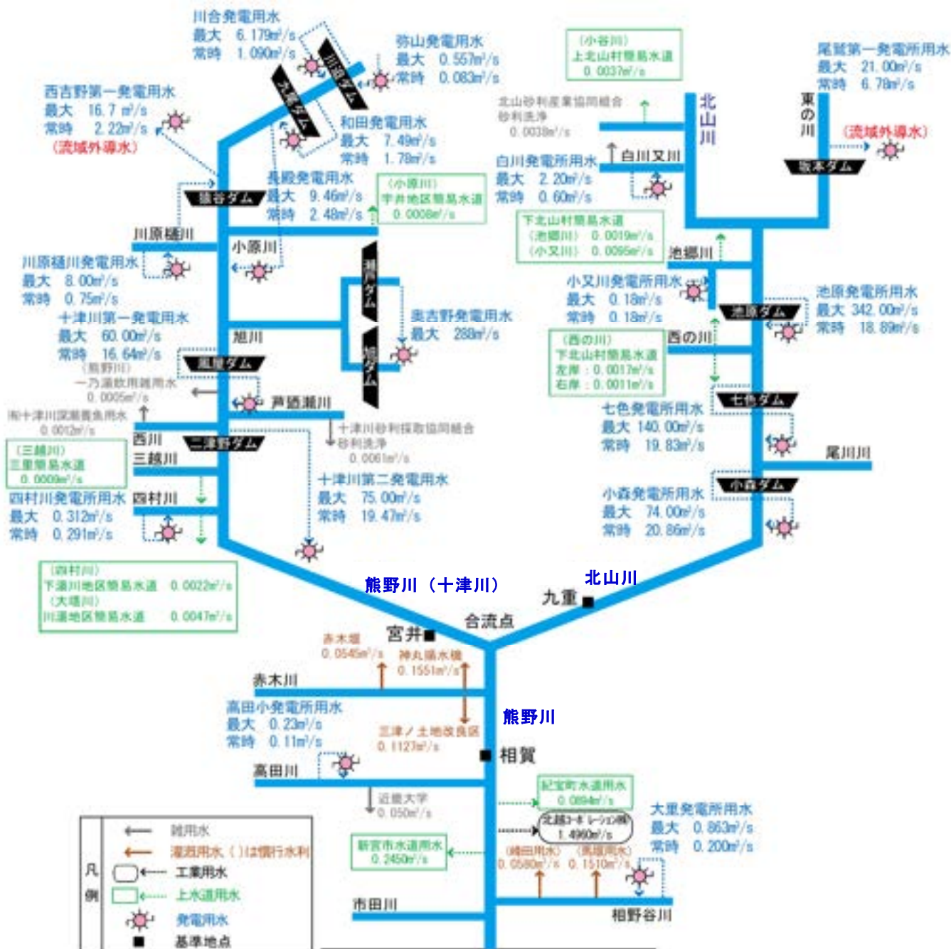
図-2.20 新宮川水系の水利模式図（令和 2 年度末時点）
