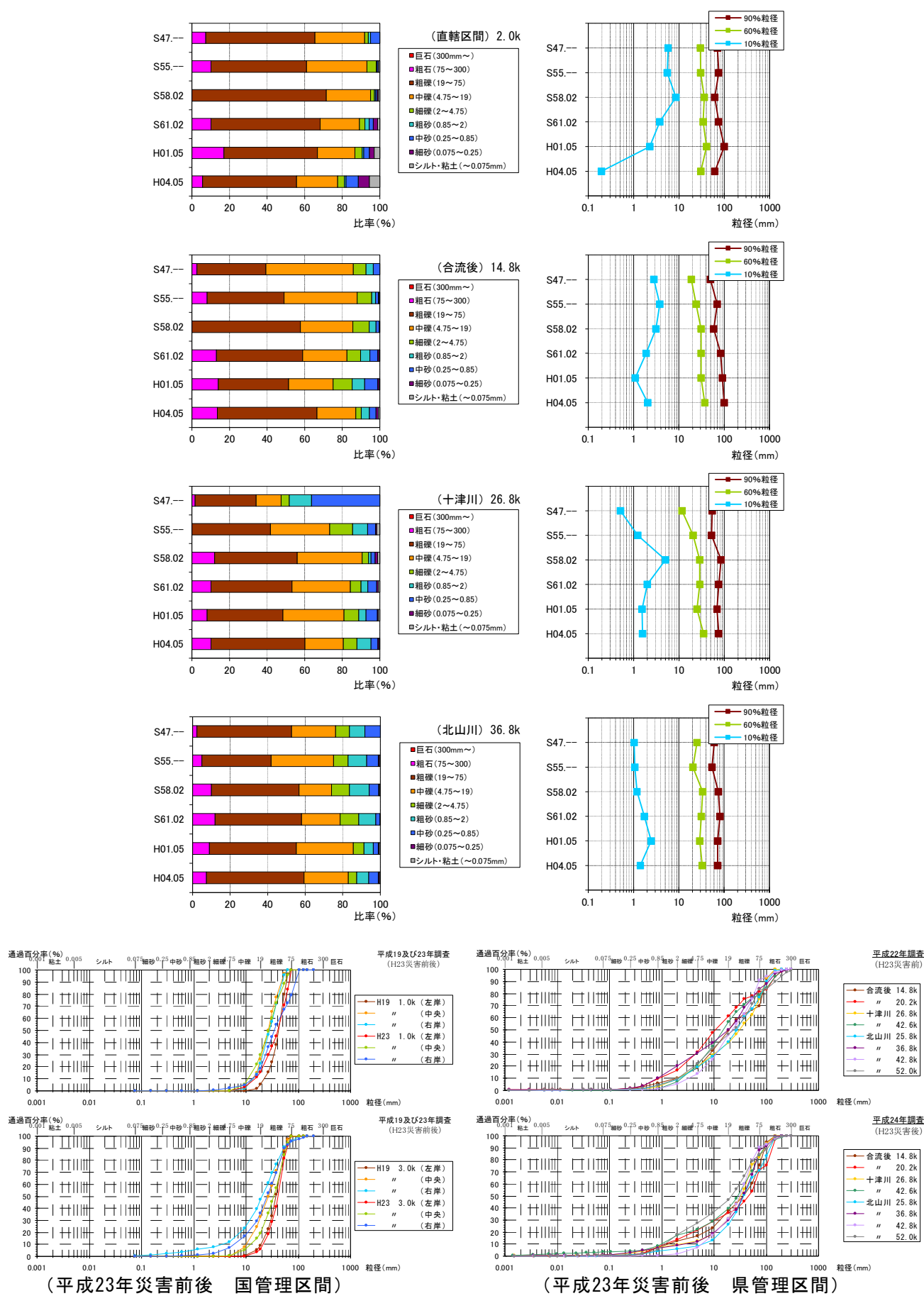
図－2.16 熊野川河床材料の経年変化
