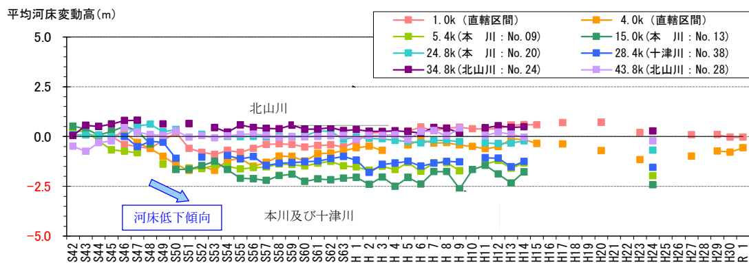
図－2.15 地点毎の平均河床の変動量（国管理区間および県管理区間）
