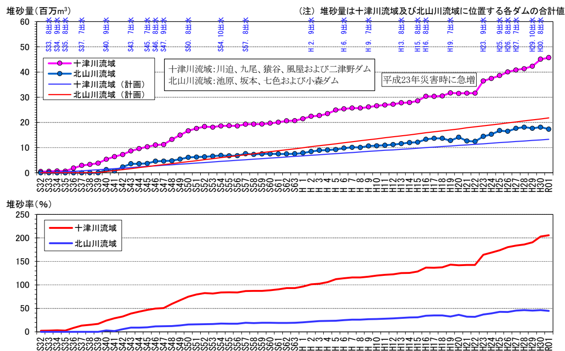
図-2.17 ダム堆砂量の経年変化
