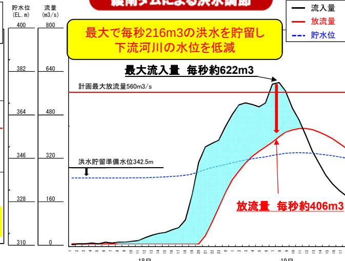
綾南ダムによる洪水調節
