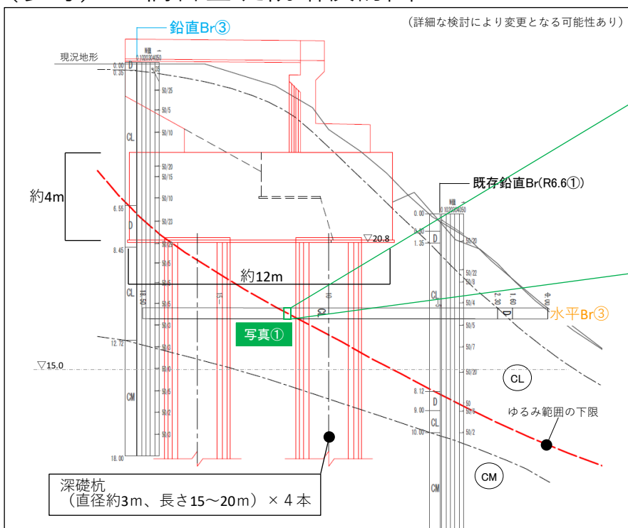
(参考) A1橋台基礎概略検討図
