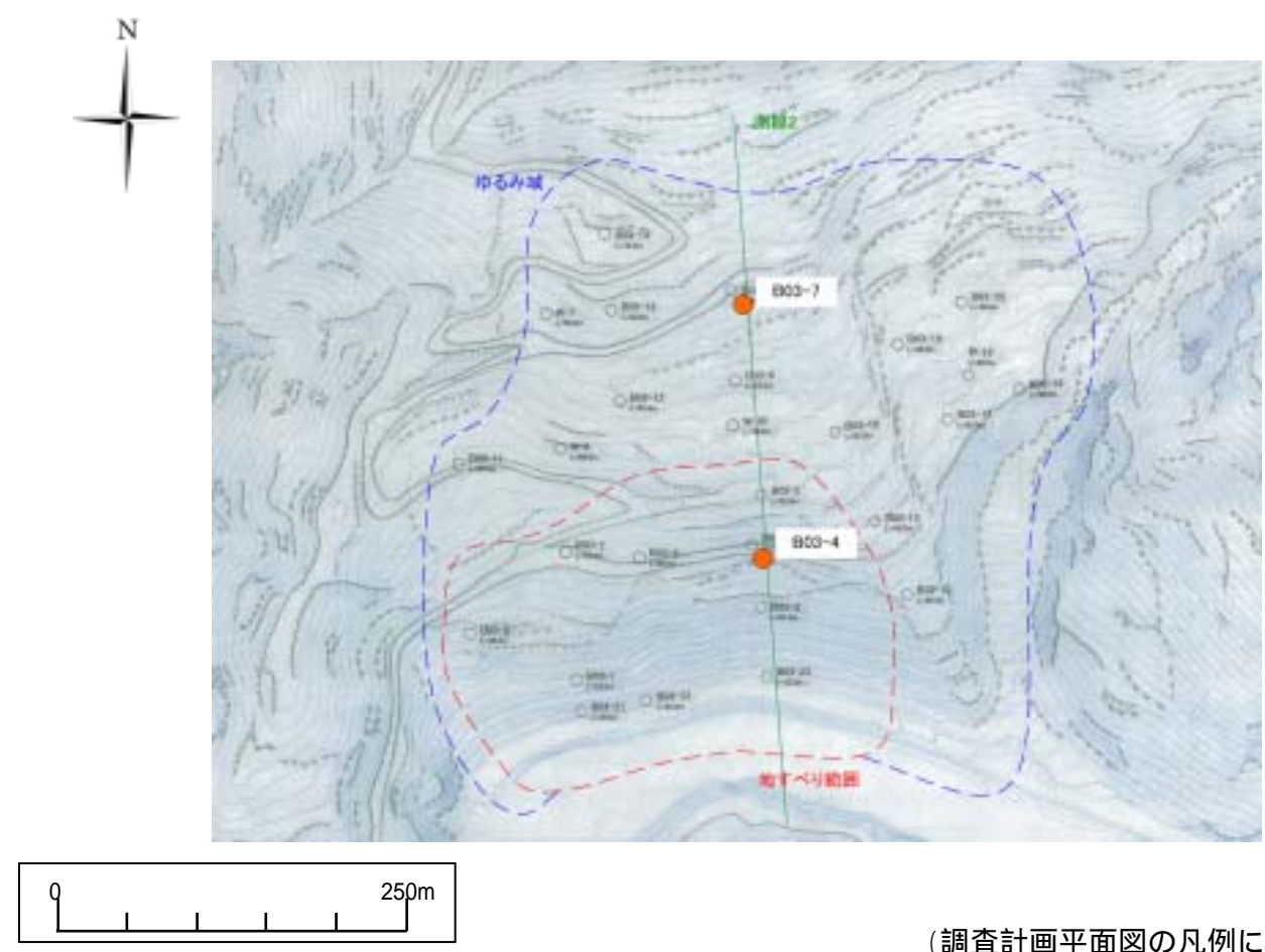
調査計画平面図・断面図
