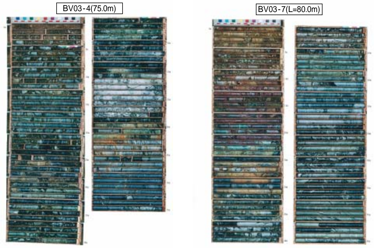
ボーリングコア写真
