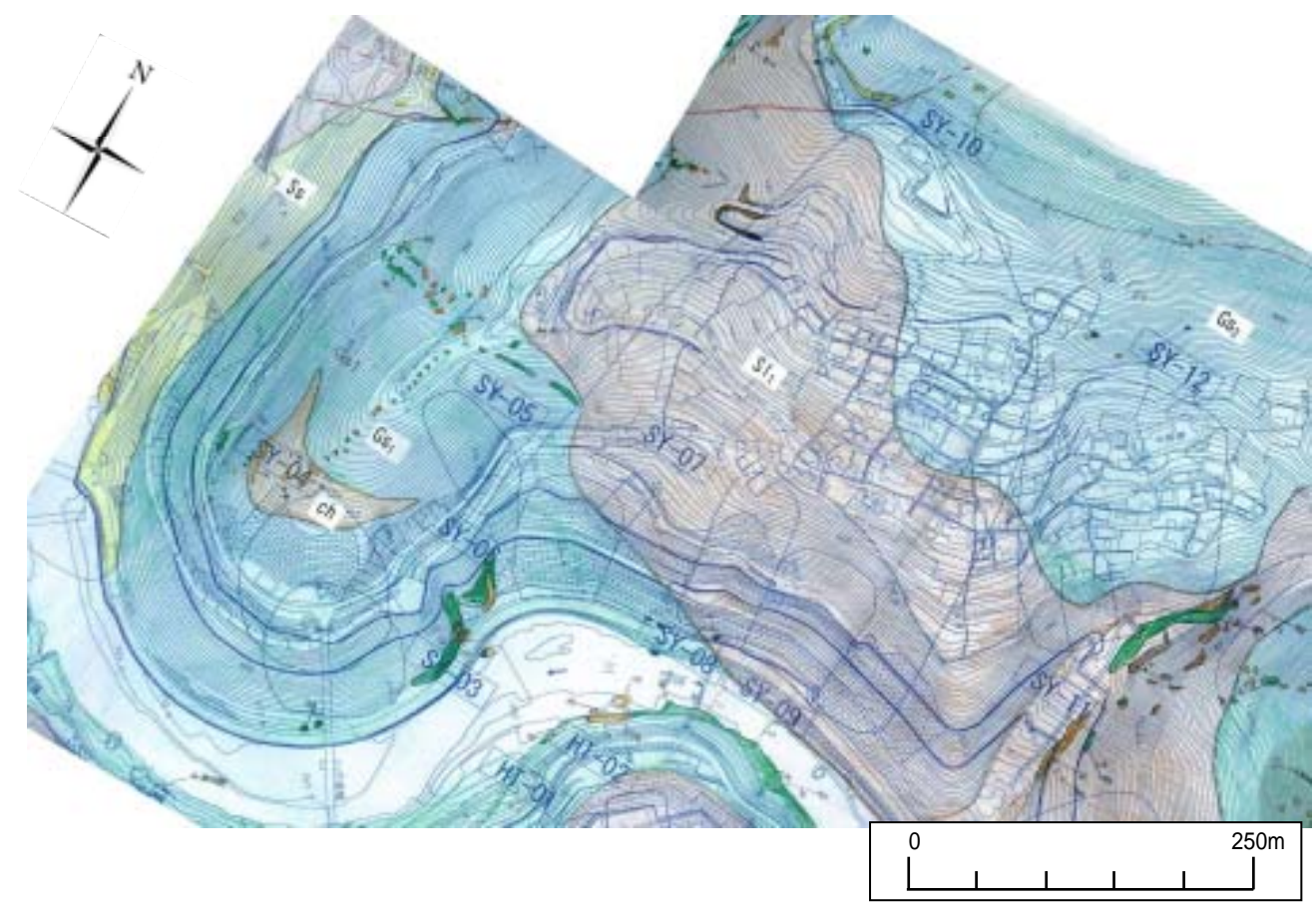
地質平面図
