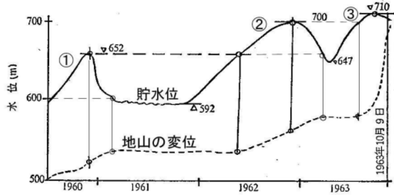
図参 - 1 バイオントダムの貯水位変化と地山変位の相関
