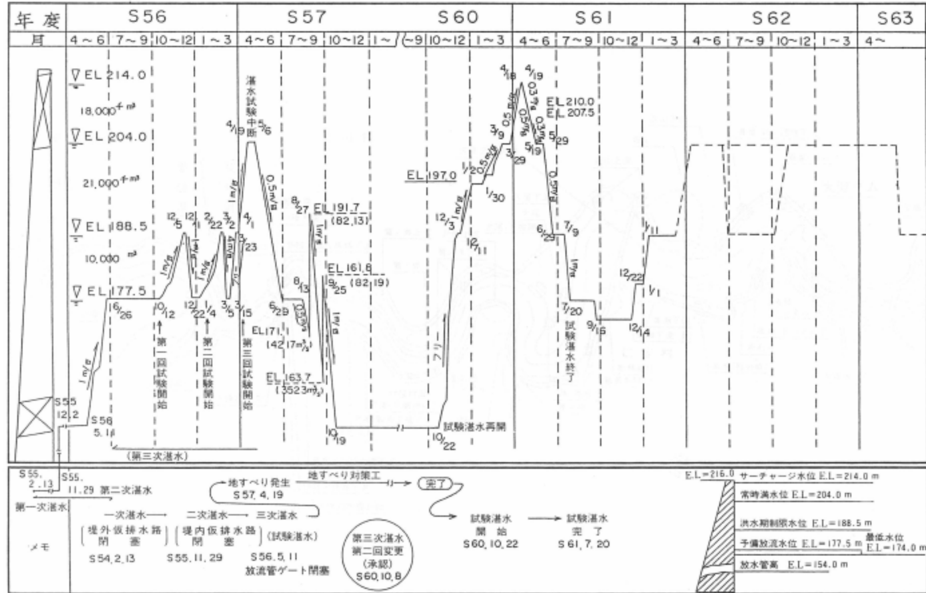
図6.1.2 大渡ダム湛水計画
