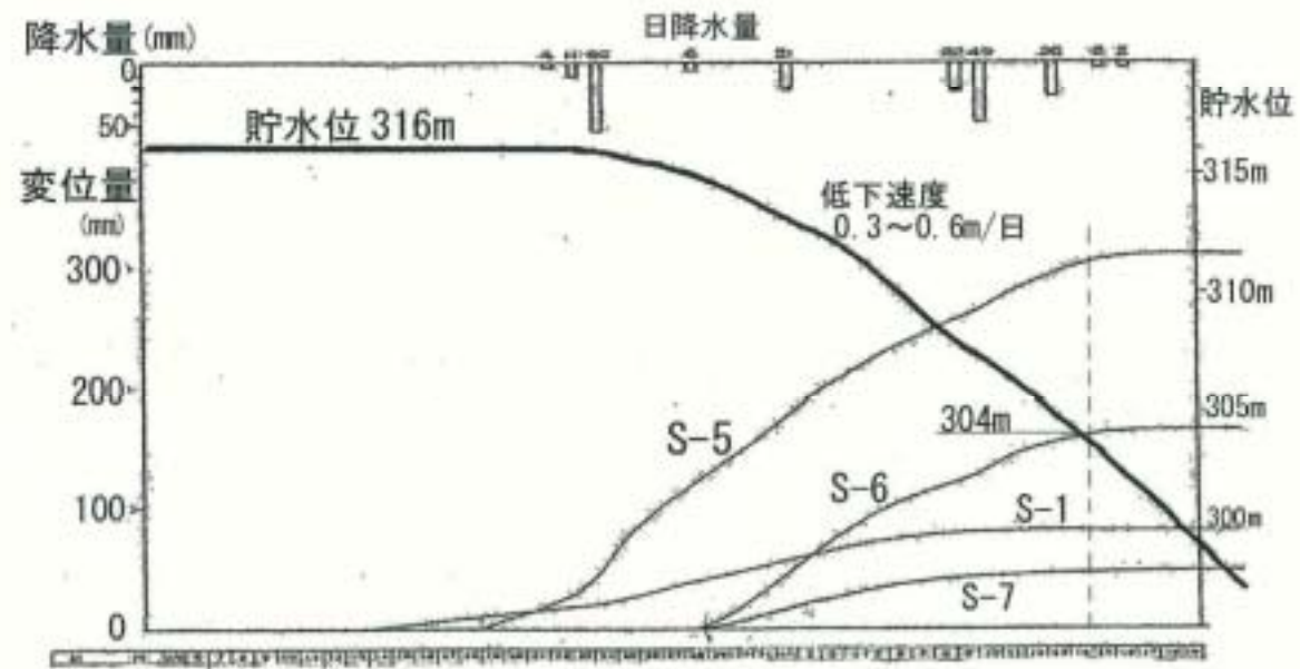
図参-3 L地区の貯水位変化と地山変位の相関
