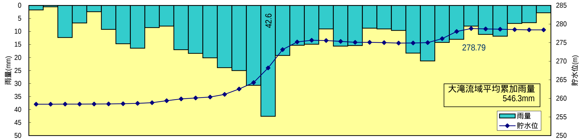
大滝流域平均雨量と大滝ダム貯水位
