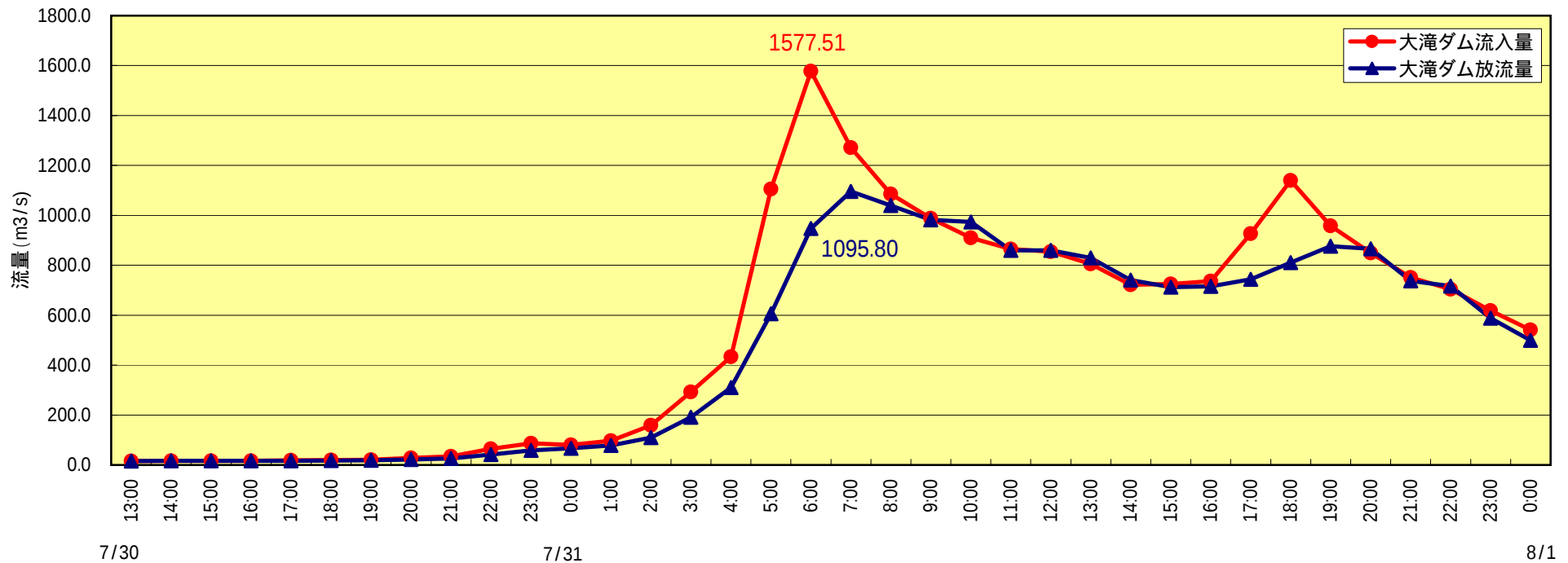
大滝ダム流入放流量
