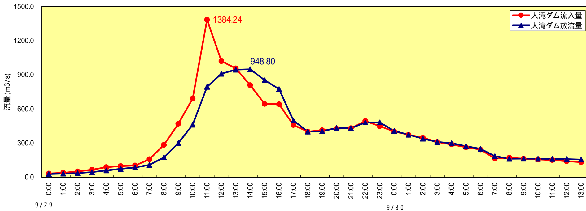
大滝ダム流入放流量
