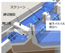
分流施設イメージ図
