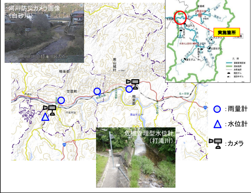
【観測設備設置位置図】
