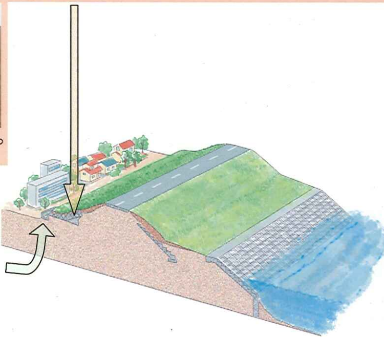
並べた石を固定するため、石の上にかゴマットを置き、中にもりとなる石を入れます。(カゴマット工)
