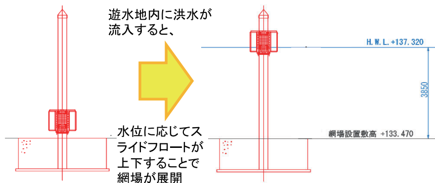
スライドフロート(平常時)
