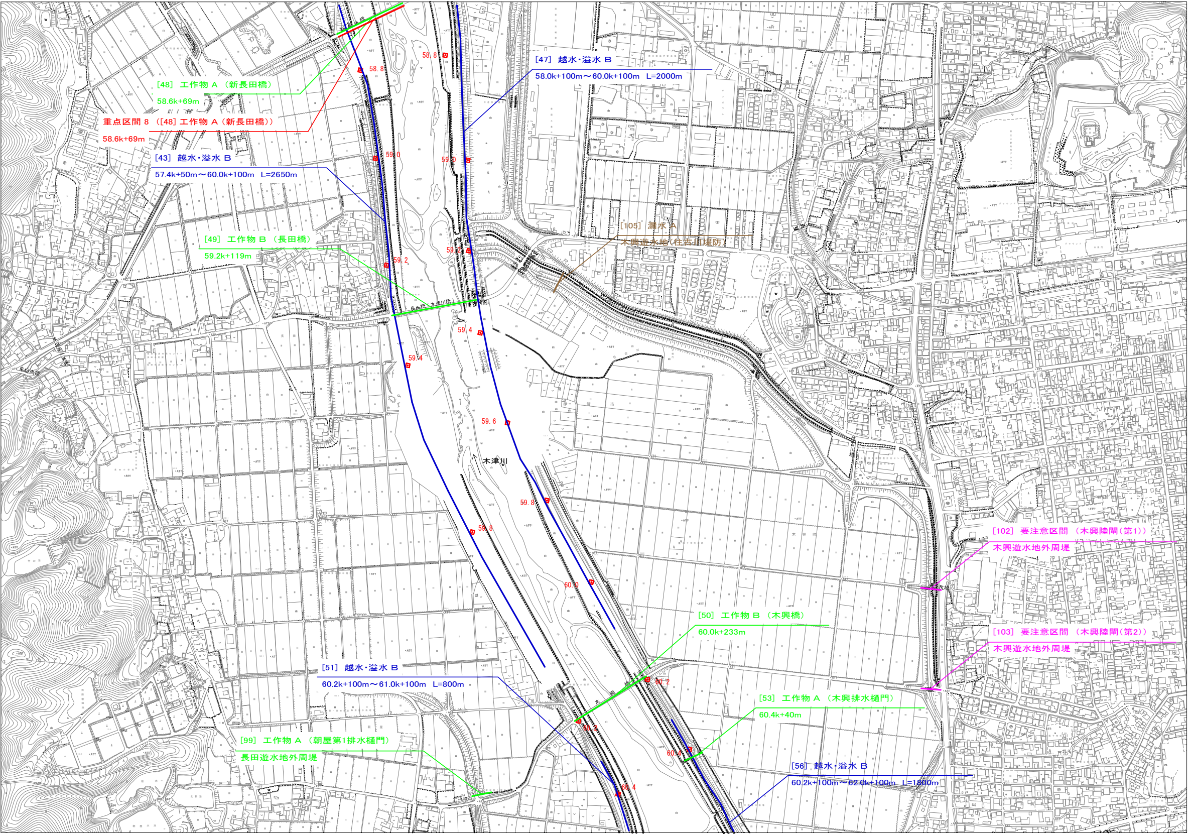
重要水防箇所 平面図（木津川8）
