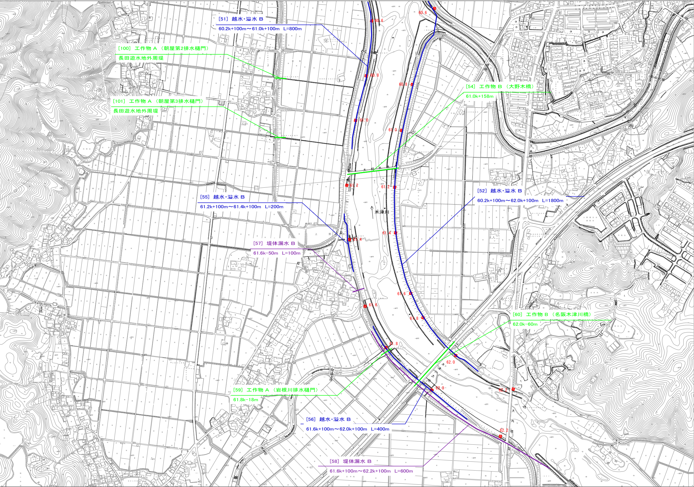
重要水防箇所 平面図（木津川9）
