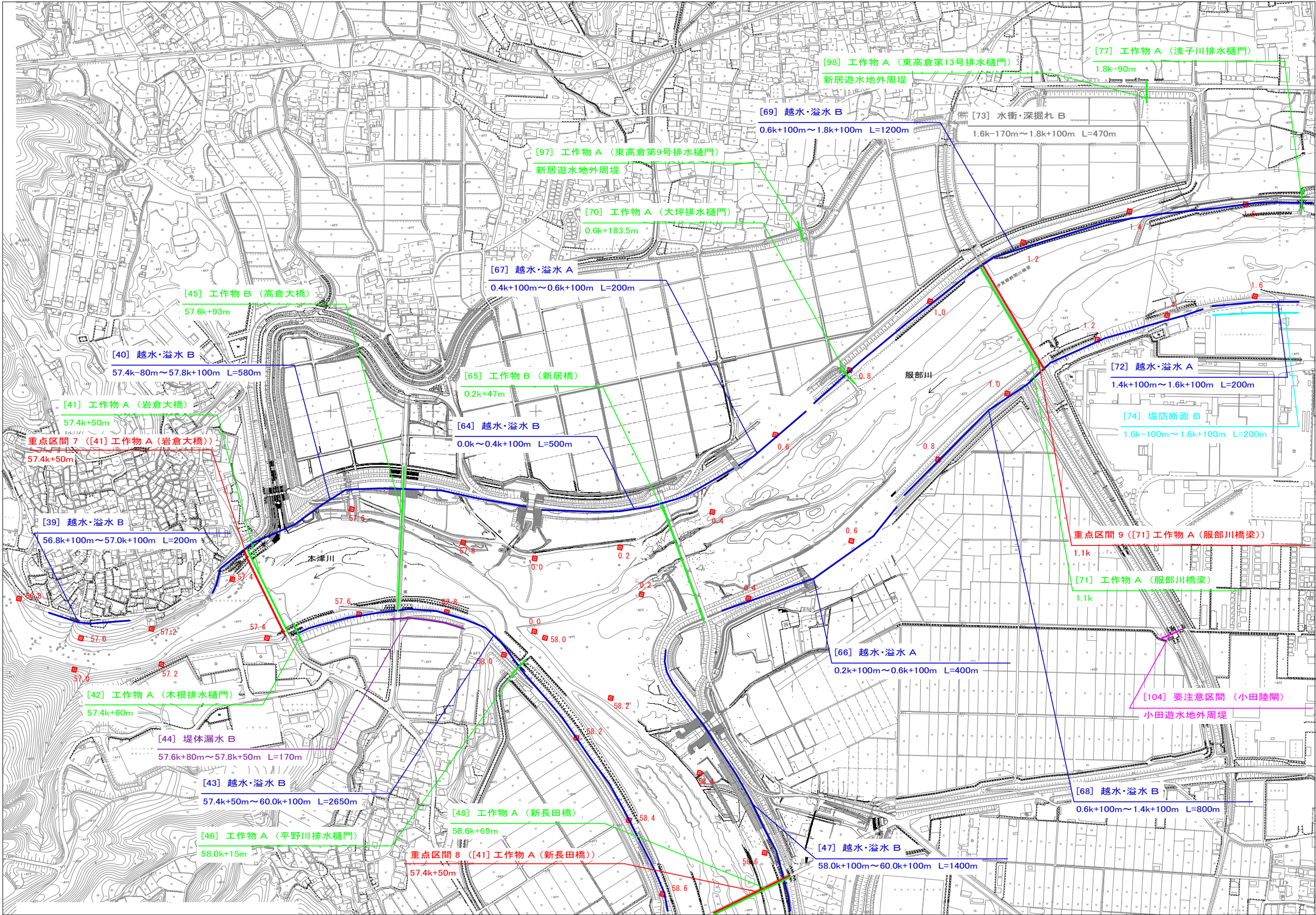
重要水防箇所 平面図（木津川7）
