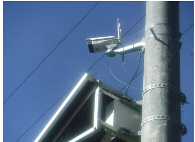
簡易型河川監視カメラ設置状況
