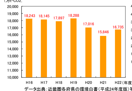
近畿圏の温室効果ガスの排出量
