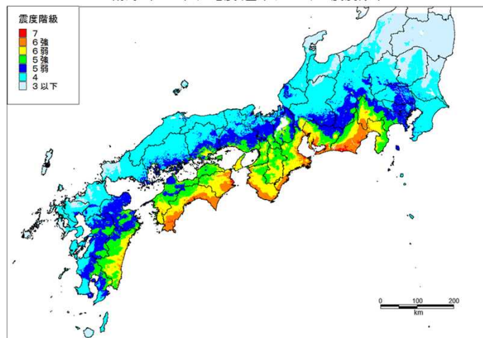
南海トラフの巨大地震(基本ケース)の震度分布
