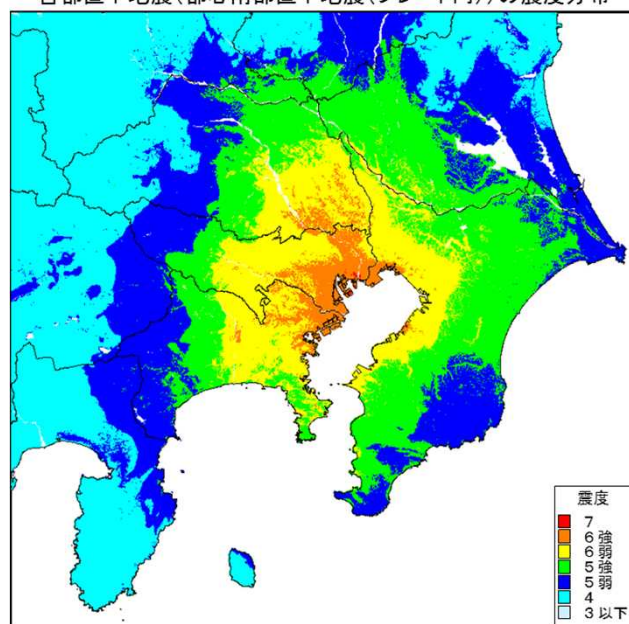
首都直下地震(都心南部直下地震(プレート内))の震度分布
