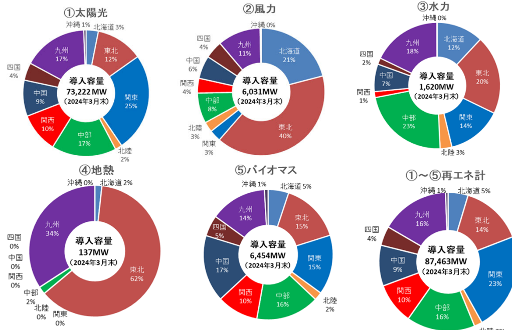
再生可能エネルギー発電設備の導入容量(2024年3月末時点)
