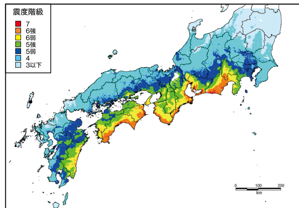
南海トラフ巨大地震(基本ケース)の震度分布
