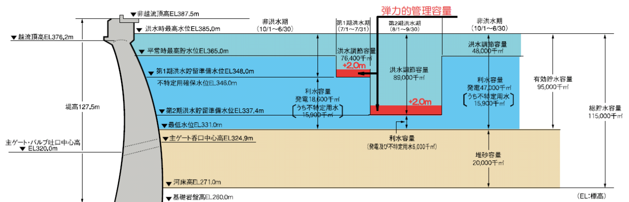
◎貯水池容量配分図
