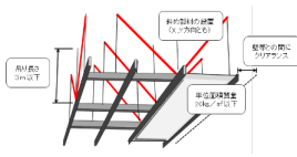
天井耐震対策
