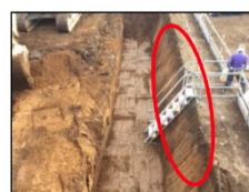
オープンカット法面整形(60° 3D)
