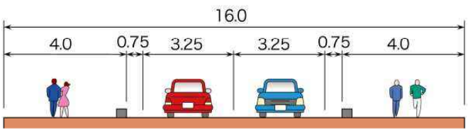
【標準断面図】
