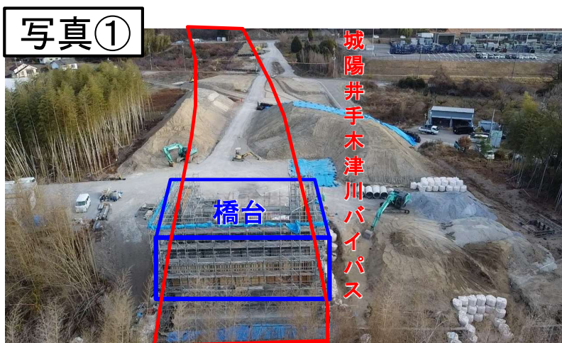
↑青谷川橋の橋梁下部工事を進めています
