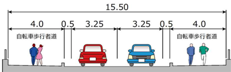
架替後の幅員構成 (単位: m)
