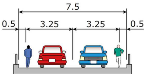
架替前の幅員構成 (単位: m)
