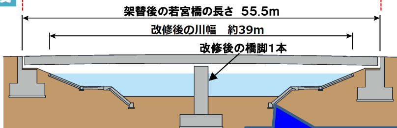
横から見た「架替後」の断面図
