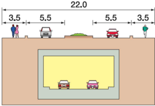
【標準断面図】
