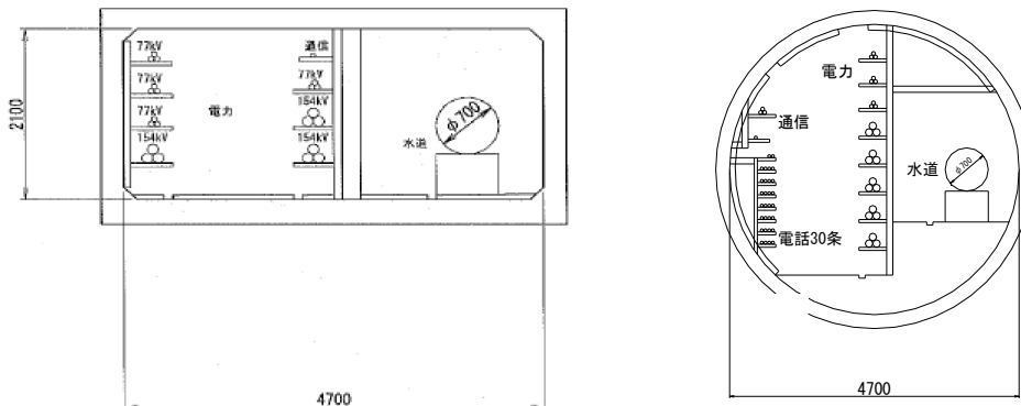
【標準断面図】
