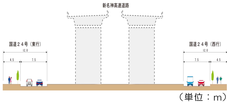
【標準断面図】
