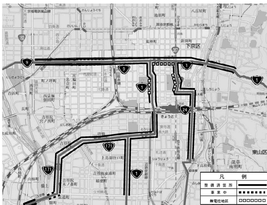
～ 電線共同溝ネットワーク図〈京都市中心部〉～
