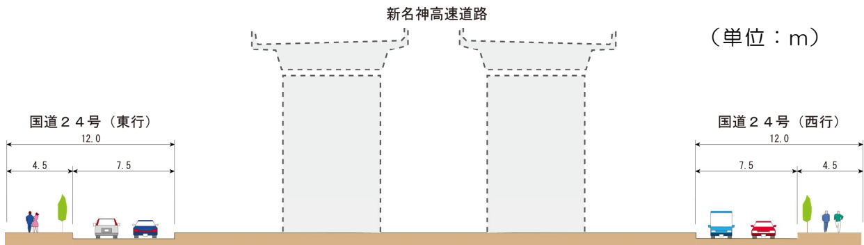
【標準断面図】
