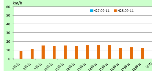
(2)大久保交差点(時間帯別旅行速度)
