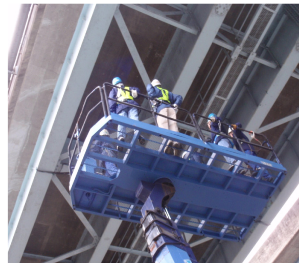
橋梁ドクターによる現地診断状況
