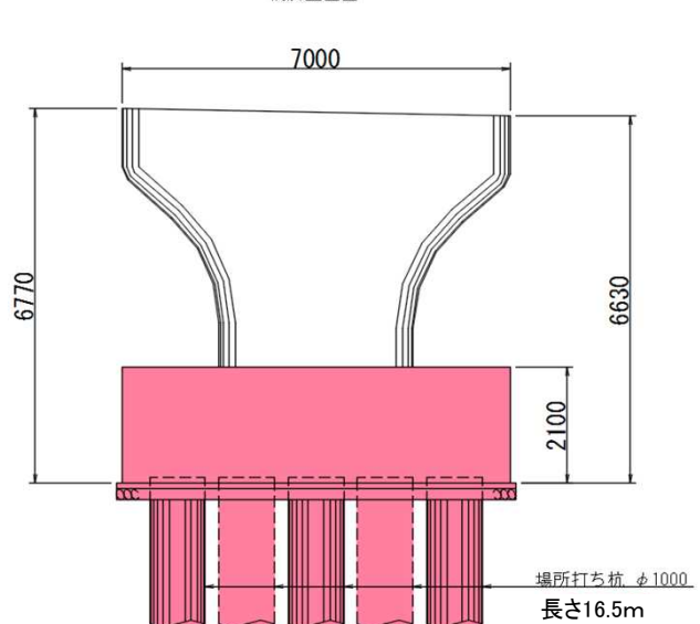
橋脚正面図
