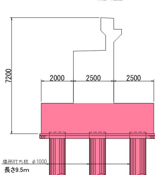
橋台断面図
