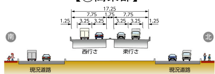
【④高架部】
