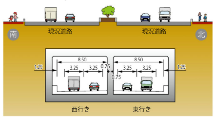
【③掘割部】
