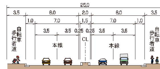
[ 標準断面図 ] 単位:m
