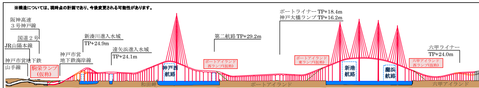
【縦断面図】
