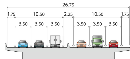
【標準断面図】 単位:m
