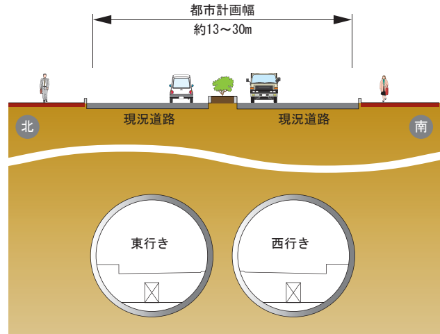
②地下式（トンネル部（シールド））
