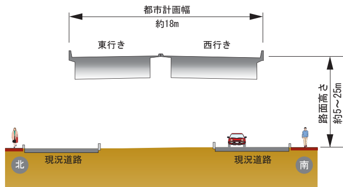
④高上式（高架部）
