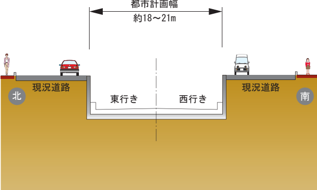
③地表式（掘割部）
