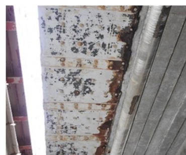
補強鋼板の腐食
