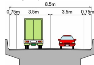
橋梁部
