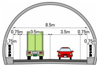
トンネル部
