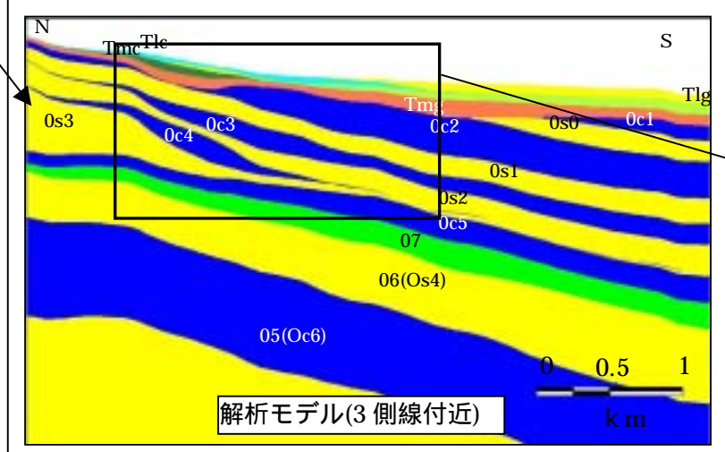
図 4-4-1 材料区分図(南北代表断面)
