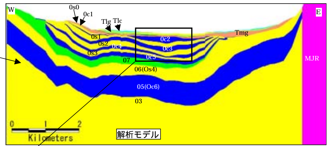
図 4-4-2 材料区分図(東西代表断面)
